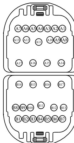
РОЗЕТОЧНЫЙ РАЗЪЕМ Электропроводка 14014
